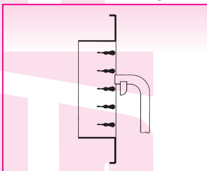
Geschwindigkeitsmessung mit Sonde 2220 A oder 6070
